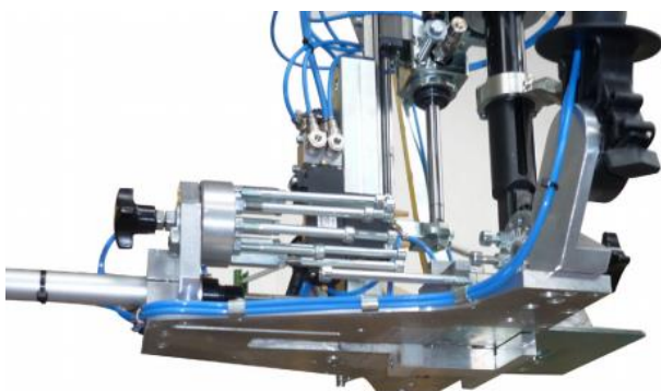
Revolveranschläge
