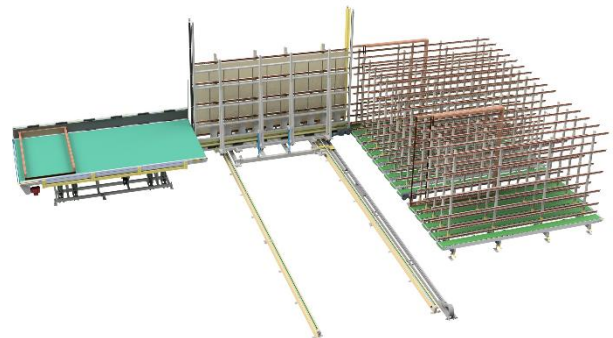
Automatischer Fachpuffer mit horizontalem Austransport
