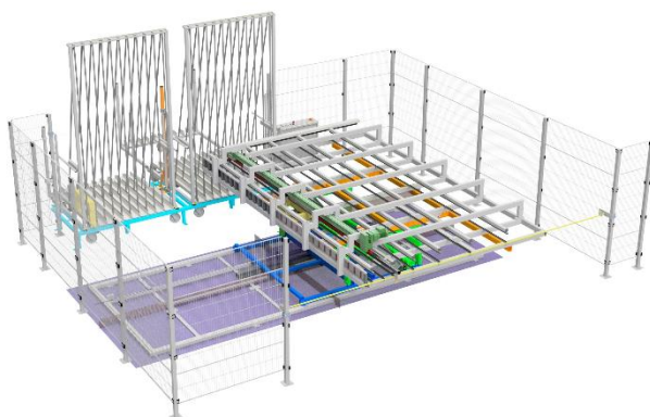
Automatische Abstellvorrichtung
