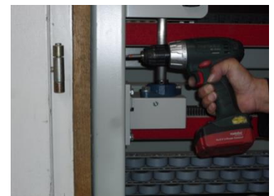
Maintien des châssis décollés de la plateforme pour le vissage de l'emballage.
